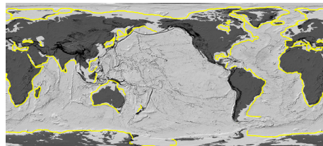
Margens Continentais Passivas.
